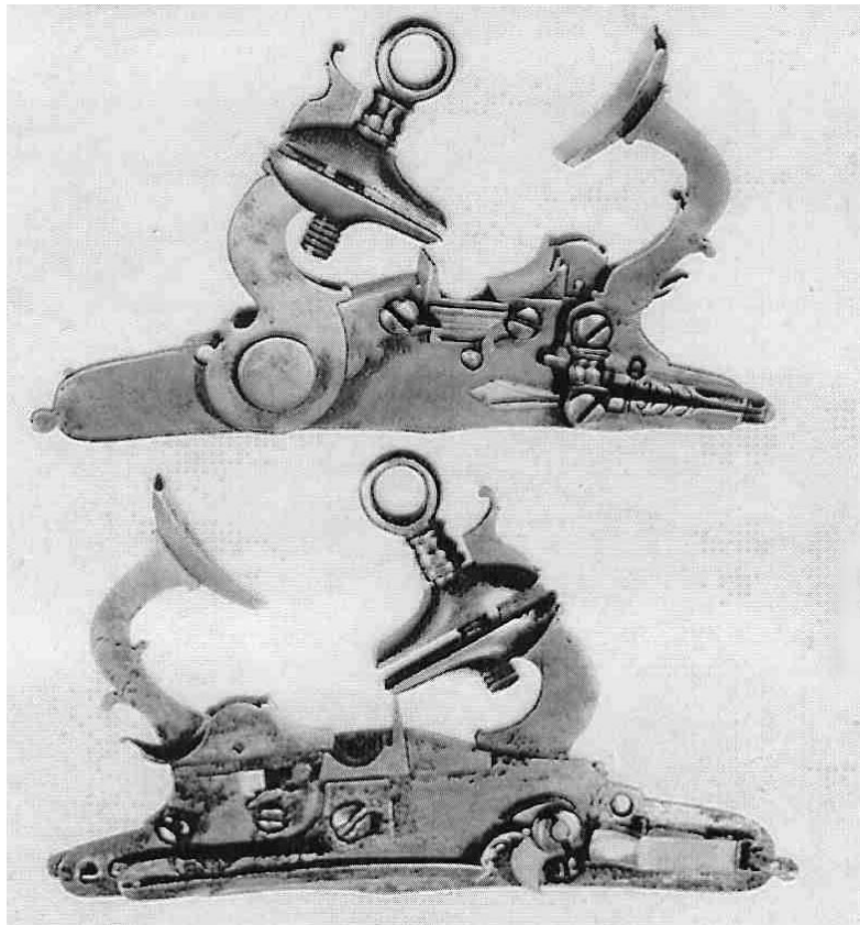
Holländisches Schnappschloss 16. – 17. Jahrhundert
