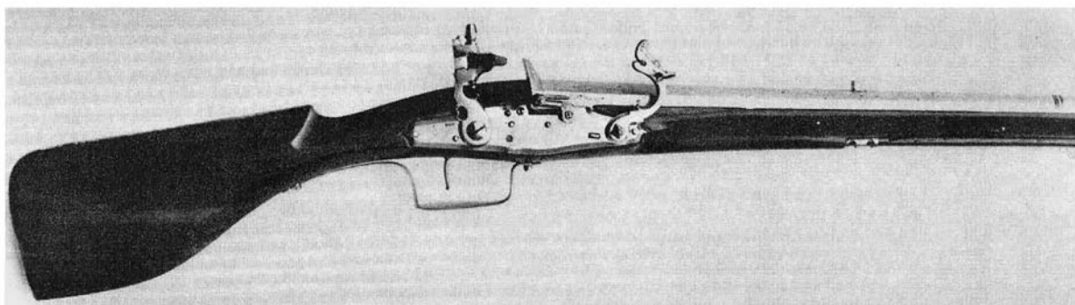
Kombiniertes Schloss (Steinschloss, Luntenschloss) Paris um 1630
