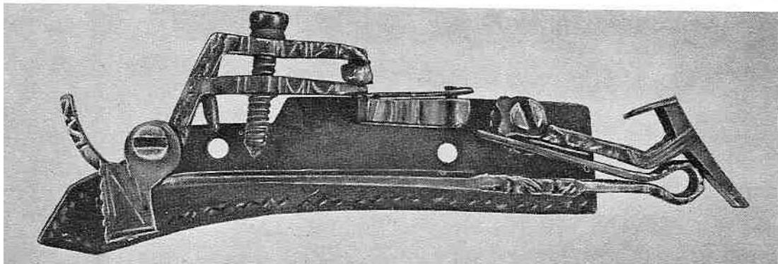
Holländisches Schnappschloss um1680
