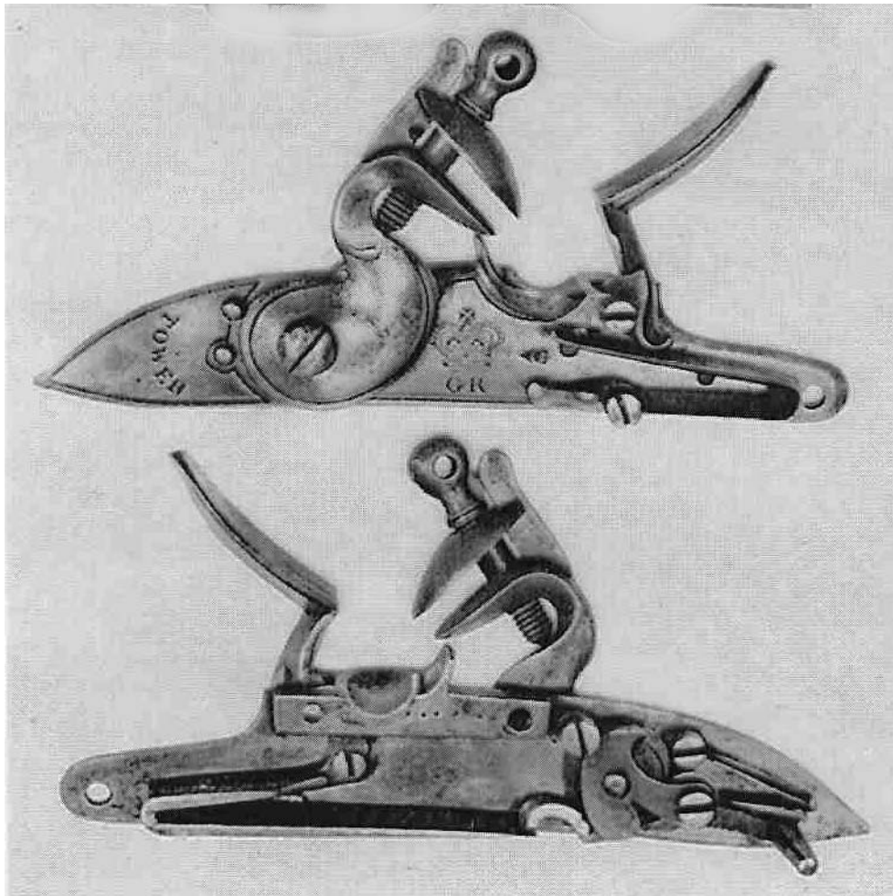
Batterieschloss England (französischer Typ) 18. Jahrhundert
